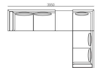
尺寸: 3950*2750*740mm
