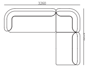
尺寸: 3260*2460*710mm
