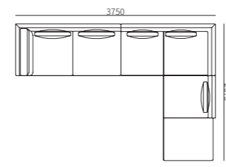
尺寸: 3750*2575*740mm
