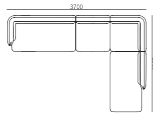
尺寸: 3700*2580*770mm
