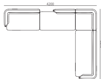
尺寸: 4200*3190*770mm
